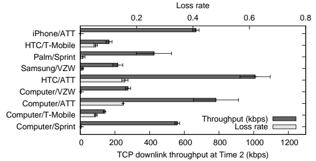
(d) Throughput and loss rate correlation (Time 2).
